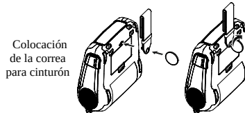
Colocación del broche de correa para cinturón
