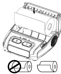
Установка бумажного рулона
